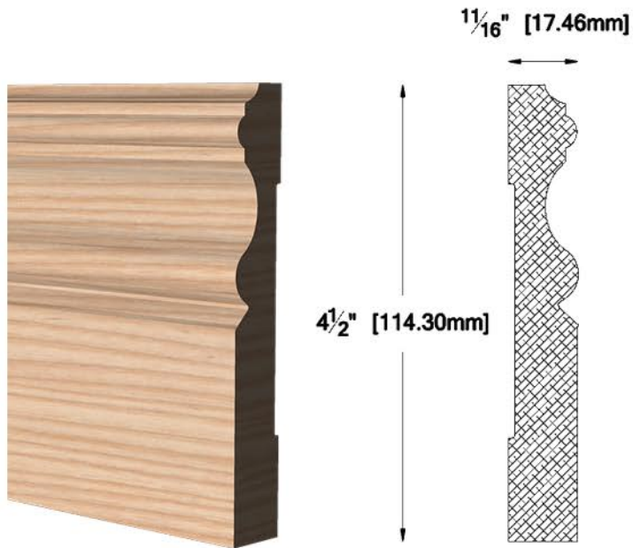
PL-4083 1 1/16" X 4 1/2" (17.46 X 114.30 mm)
