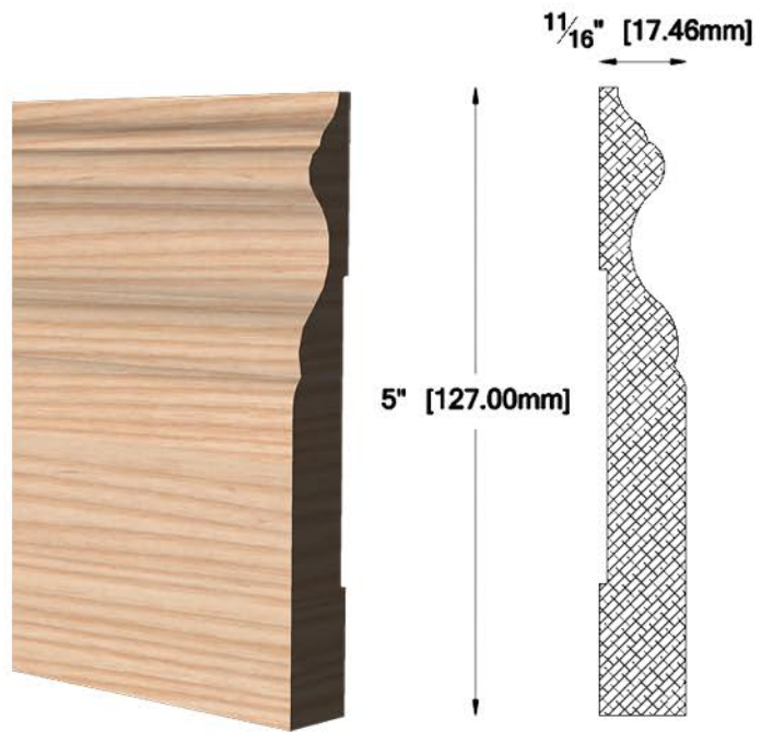
PL-5010 11/16" X 5" (17.46 X 127.00 mm)
