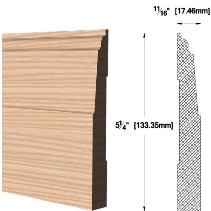
PL-5005 1 1/16" X 5 1/4" (17.46 X 133.35 mm)
