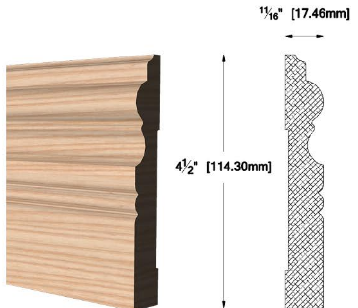
PL-4024 1 1/16" X 4 1/2" [17.46 X 114.30 mm]
