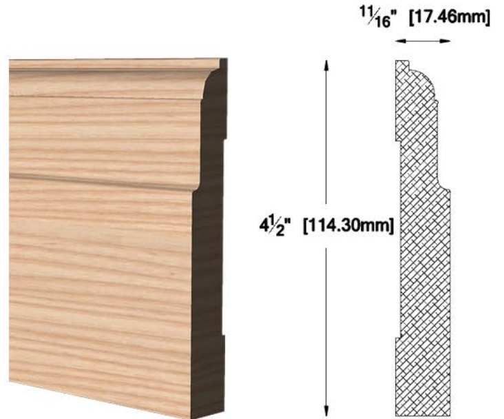
PL-4002 1 1/16" X 4 1/2" [17.46 X 114.30 mm]
