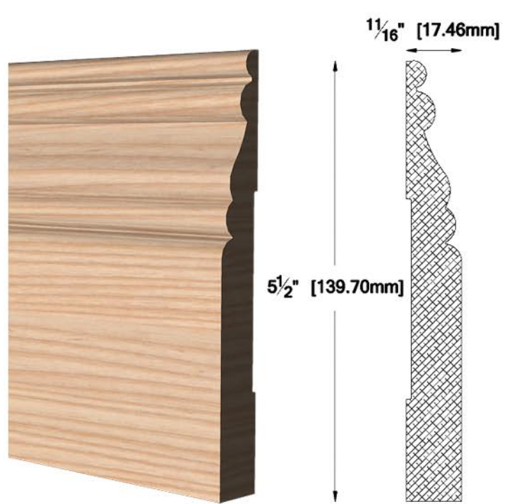
PL-5006 1 1/16" X 5 1/2" (17.46 X 139.70 mm)
