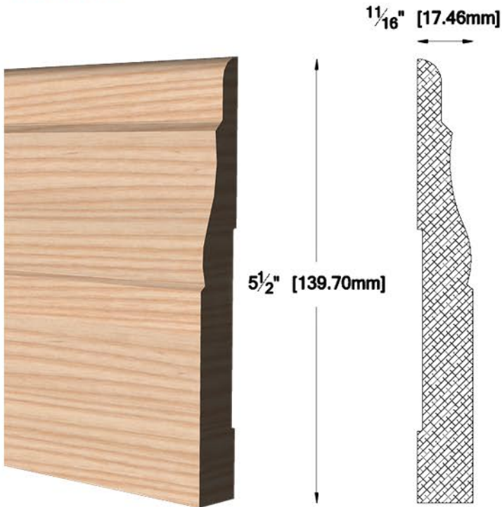
PL-5003 1 1/16" X 5 1/2" (17.46 X 139.70 mm)
