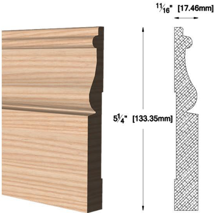
PL-5007 11/16" X 5 1/4" (17.46 X 133.35 mm)
