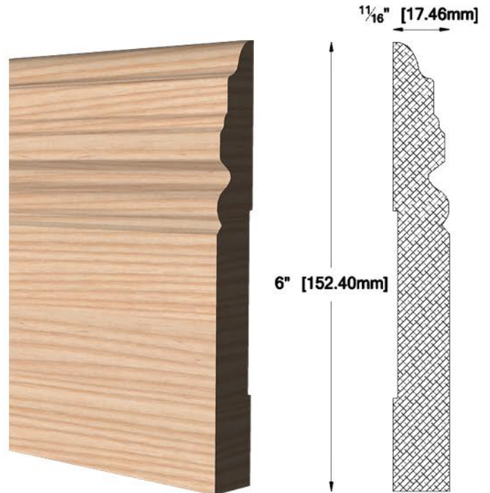
PL-5020 1 1/16" X 6" (17.46 X 152.40 mm)
