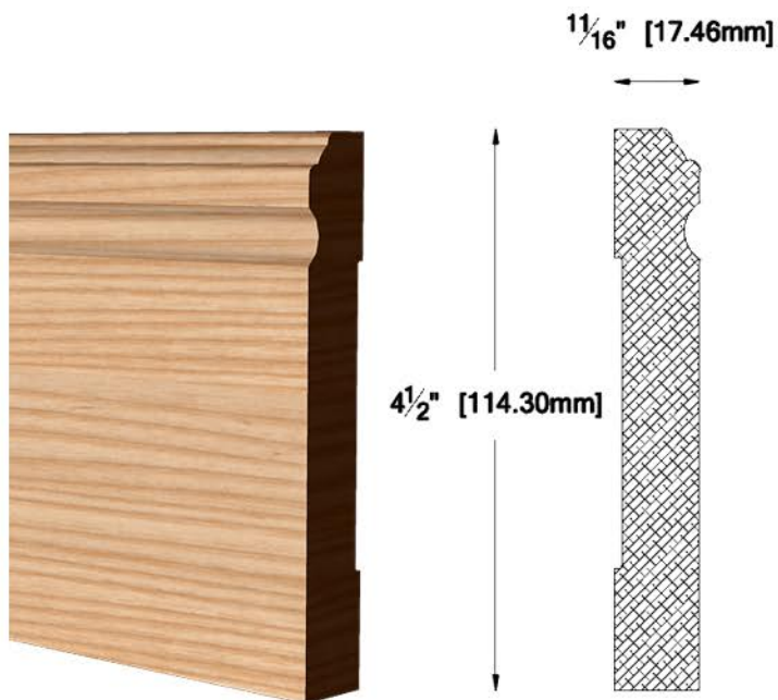
PL-4531 1 1/16" X 4 1/2" (17.46 X 114.30 mm)
