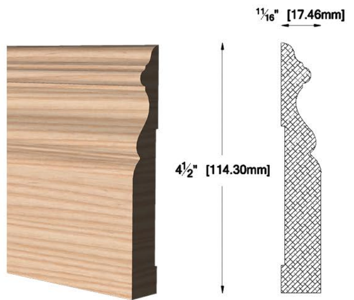
PL-4500 1 1/16" X 4 1/2" (17.46 X 114.30 mm)
