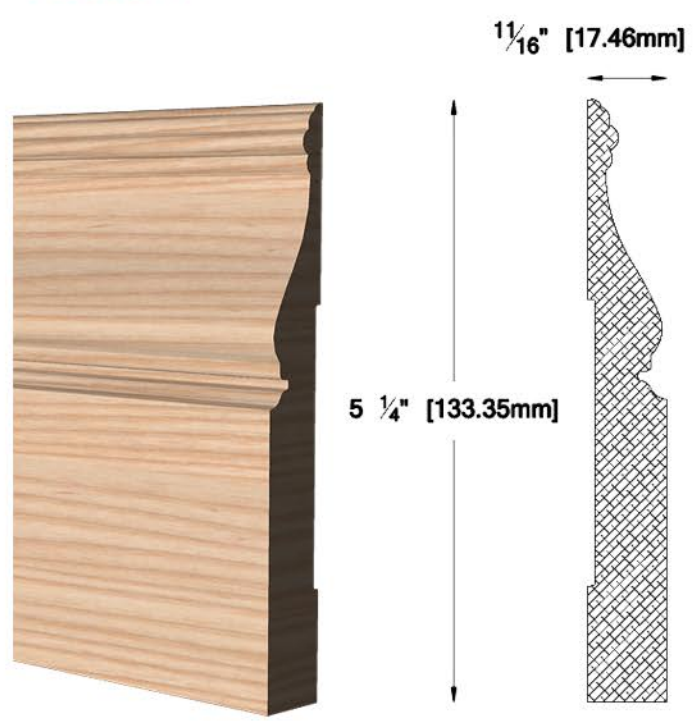
PL-5004 1 1/16" X 5 1/4" (17.46 X 133.35 mm)
