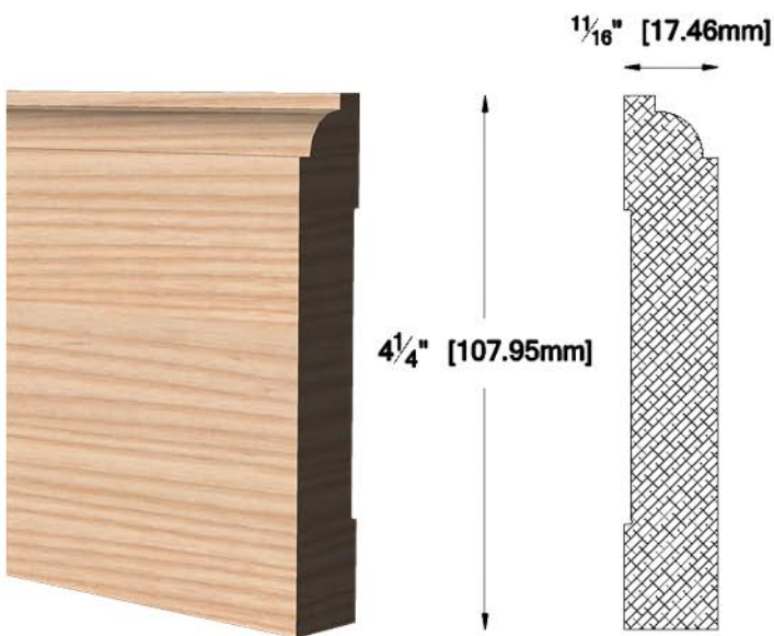
PL-4011 1 1/16" X 4 1/4" [17.46 X 107.95 mm]
