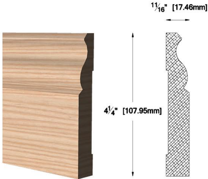
PL-4001 1 1/16" X 4 1/4" [17.46 X 107.95 mm]
