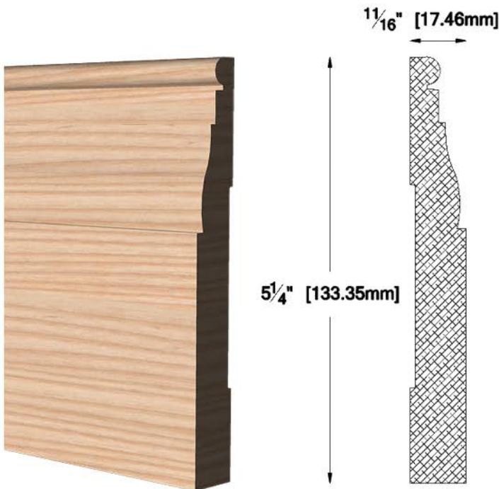
PL-5009 11/16" X 5 1/4" (17.46 X 133.35 mm)
