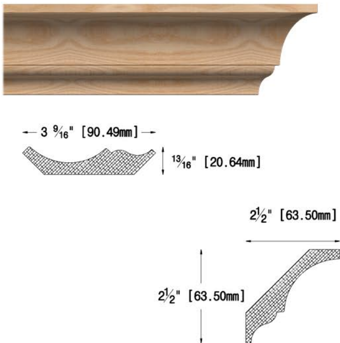
OG-4028 13/16" X 3 9/16" (20.64 X 90.49 mm)
