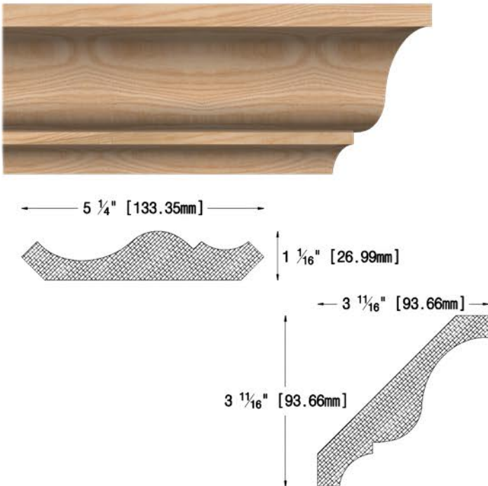
OG-5026 1 1/16" X 5 1/4" (26.99 X 133.35 mm)
